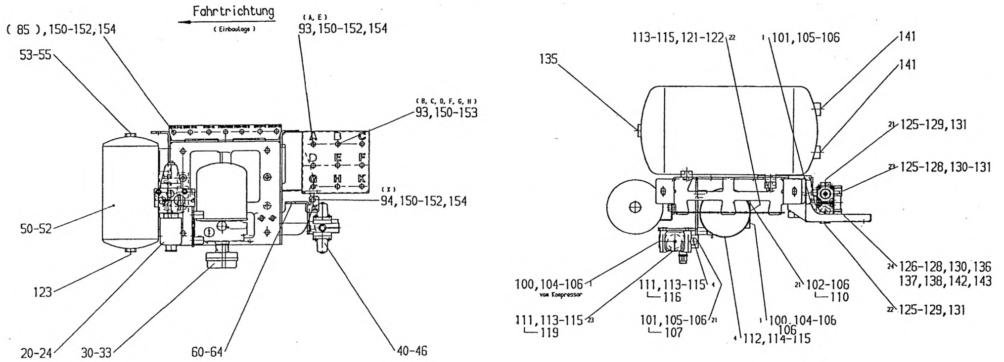
Bestückung - Druckschalter
