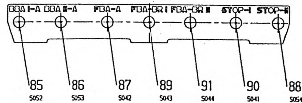
Bestückung - Druckschalter
